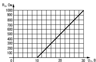
Рисунок 5.19 – График зависимости R_H(U_n)
