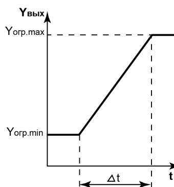
Рисунок 7.11 – Ограничение скорости изменения сигнала
