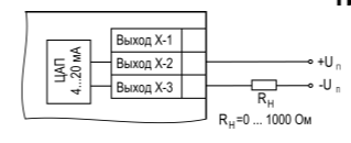
Рисунок 24 – Схема подключения нагрузки к ВУ типа И
