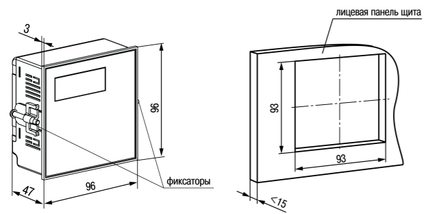
Рисунок 6 – Габаритные размеры корпуса Щ11
