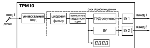
Рисунок 28 – Функциональная схема прибора
