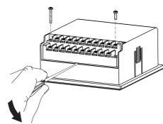
Рисунок 8 – «Быстрая» замена прибора
