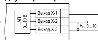
Рисунок 27 – Схема подключения нагрузки к ВУ типа У
