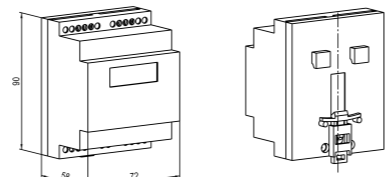
Рисунок 9 – Габаритные размеры корпуса Д
