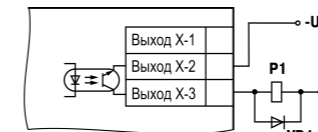
Рисунок 20 – Схема подключения нагрузки к ВУ типа К
