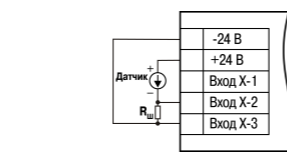
Рисунок 17 – Схема подключения пассивного датчика с питанием от прибора
