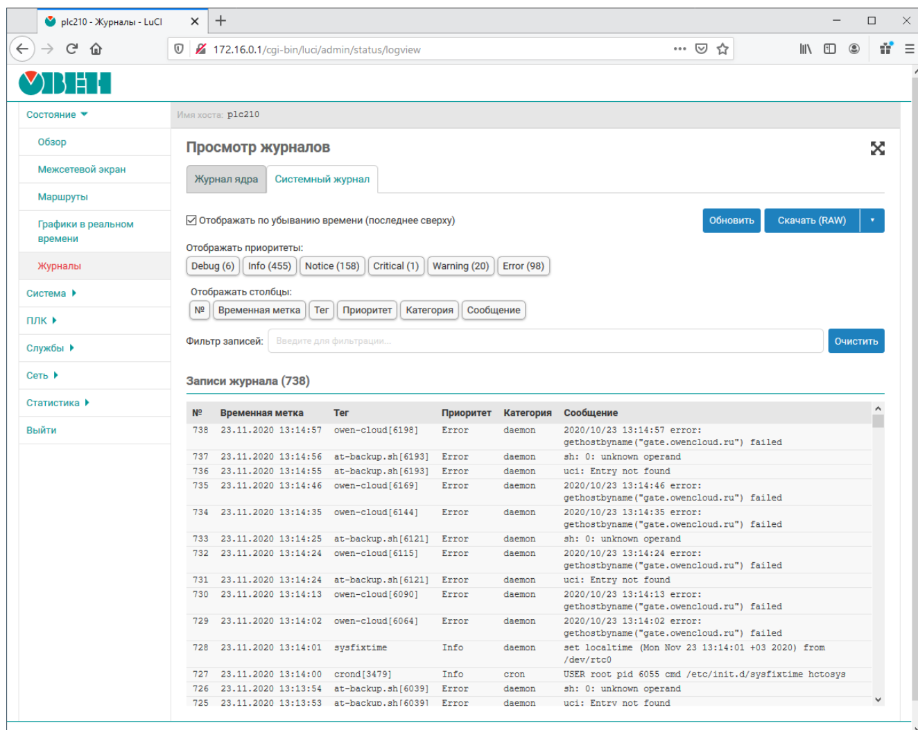
Рис. 3-21: Вкладка «Системный журнал»
