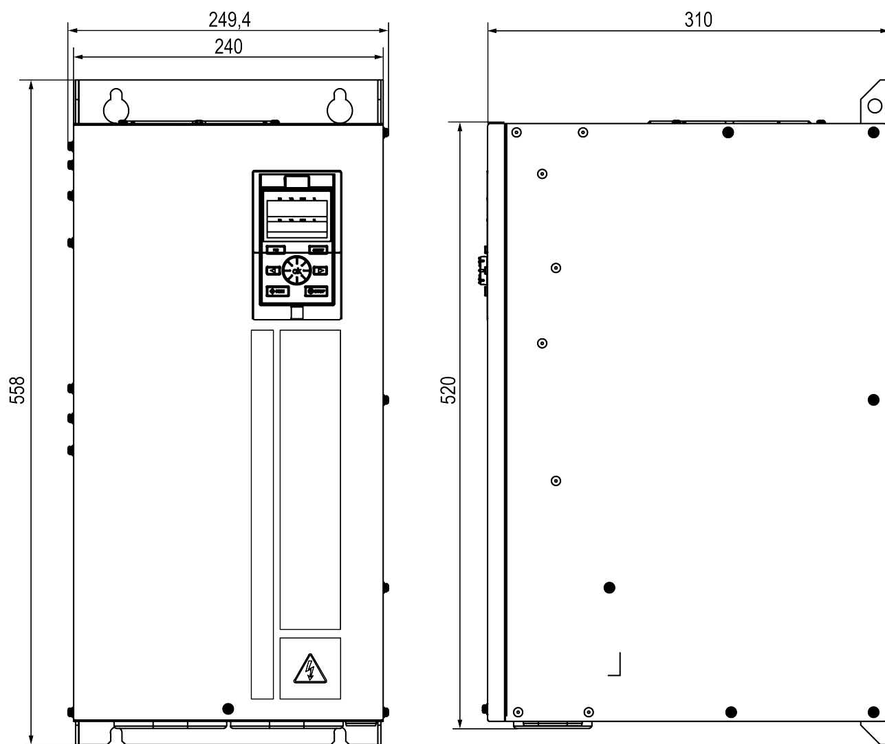
Рисунок 7.6 – Габаритные размеры прибора в корпусе типоразмера 6
