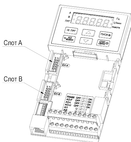
Рисунок 8.4 – Расположение разъемов для подключения плат расширения
