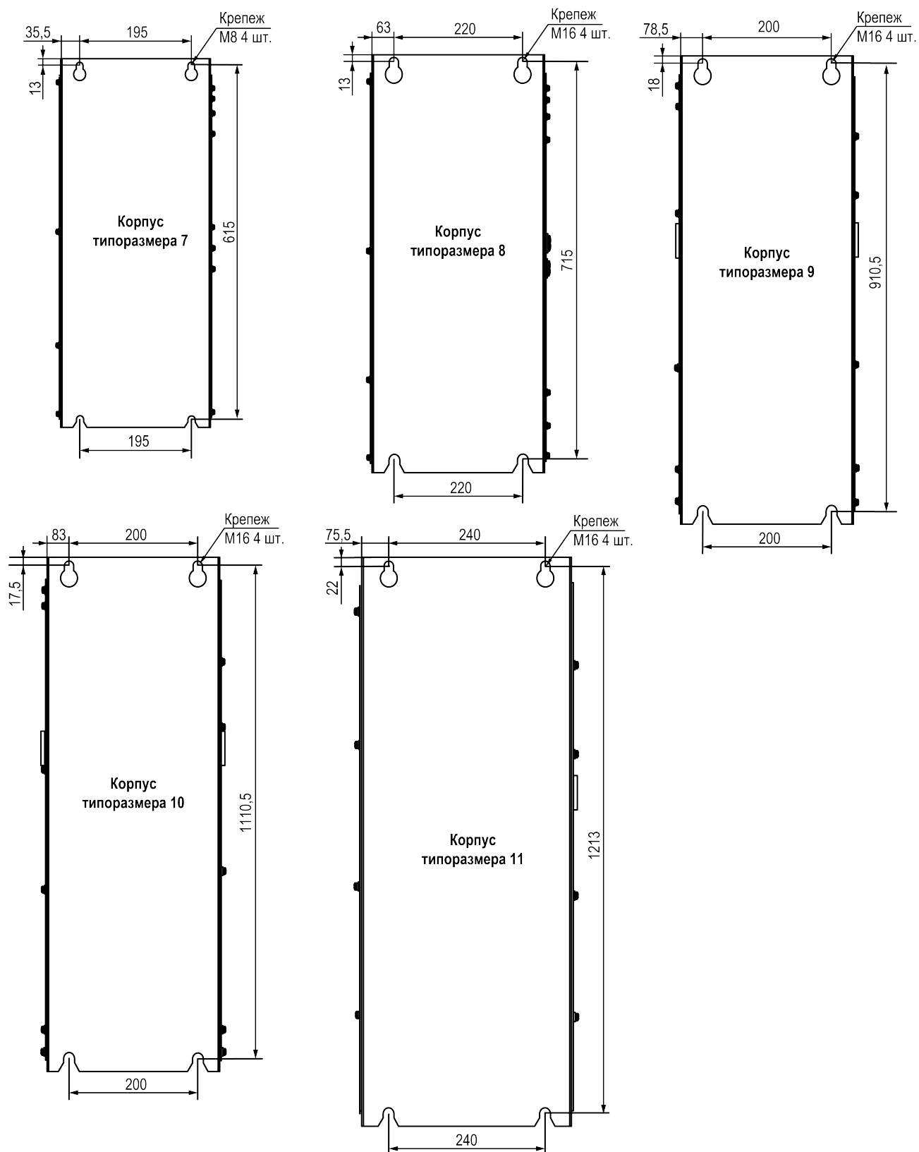
Рисунок 7.13 – Присоединительные размеры для корпусов типоразмеров 7–11
