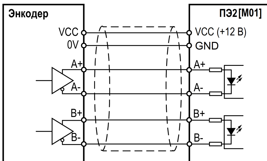
Рисунок 8.14 – Схема подключения энкодера с дифференциальным выходом
