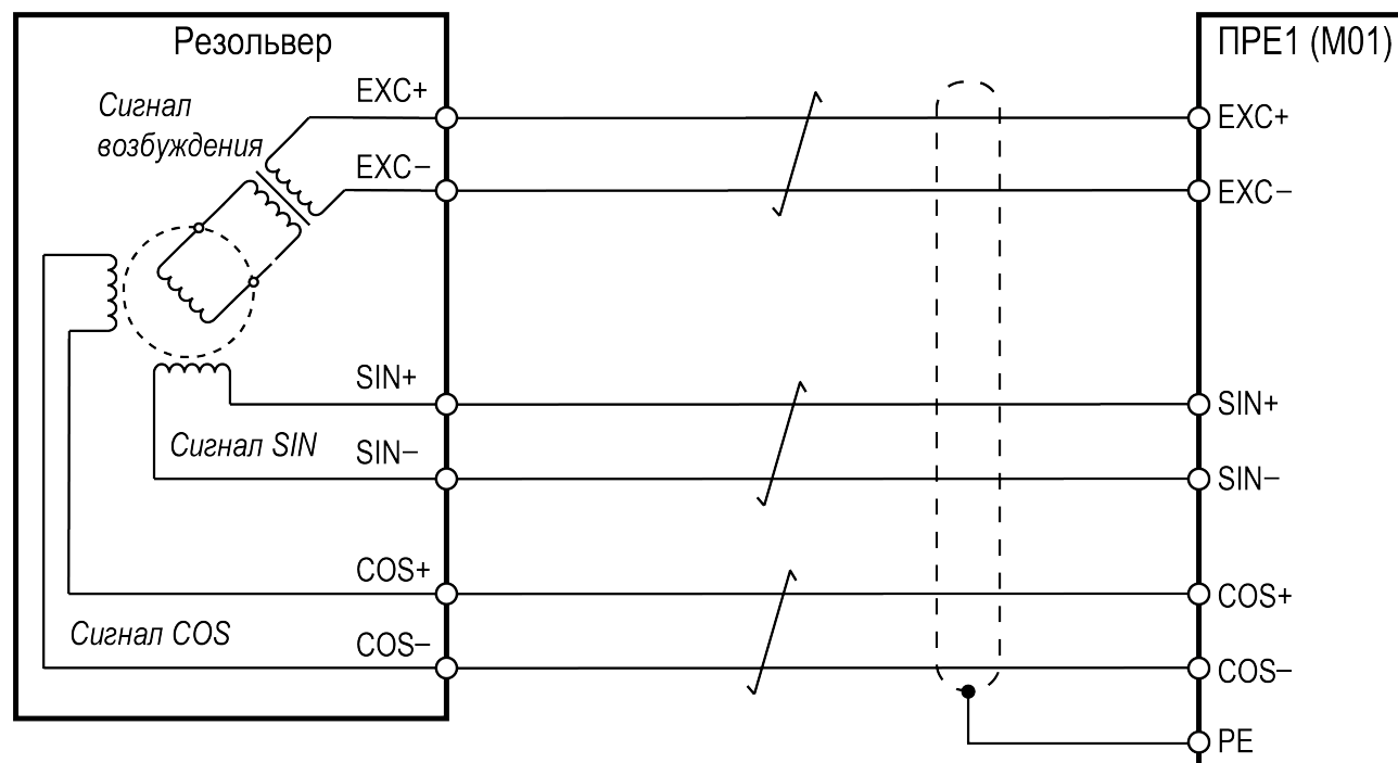
Рисунок 8.17 – Схема подключения резольвера
