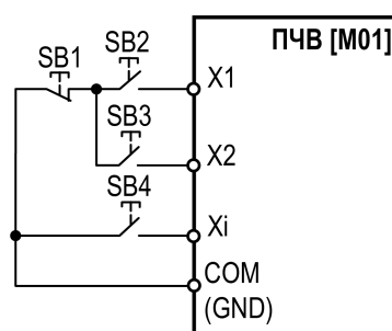
Рисунок 8.8 – Трехпроводная схема управления 1 (F05.20 = 2)
