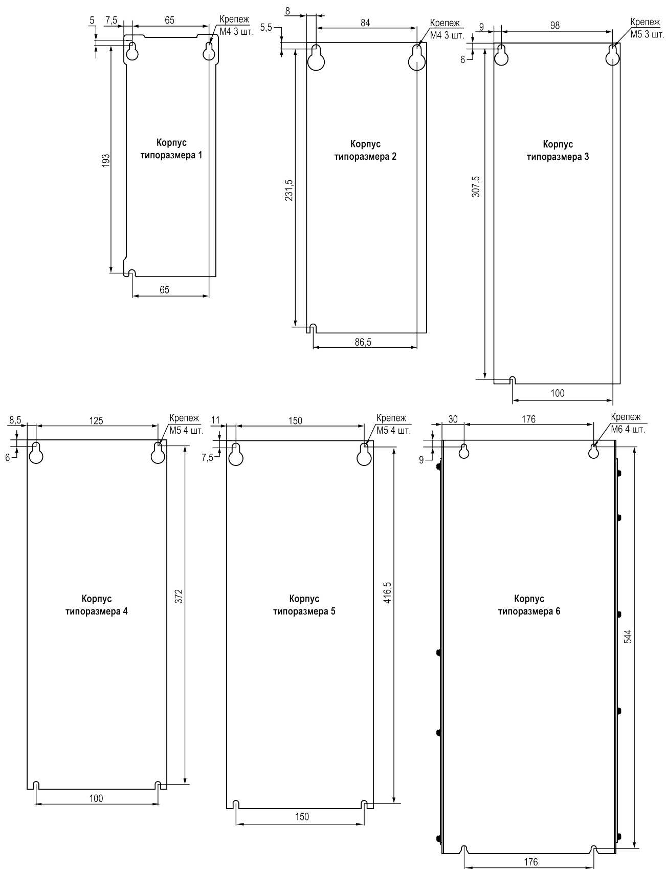
Рисунок 7.12 – Присоединительные размеры для корпусов типоразмеров 1–6
