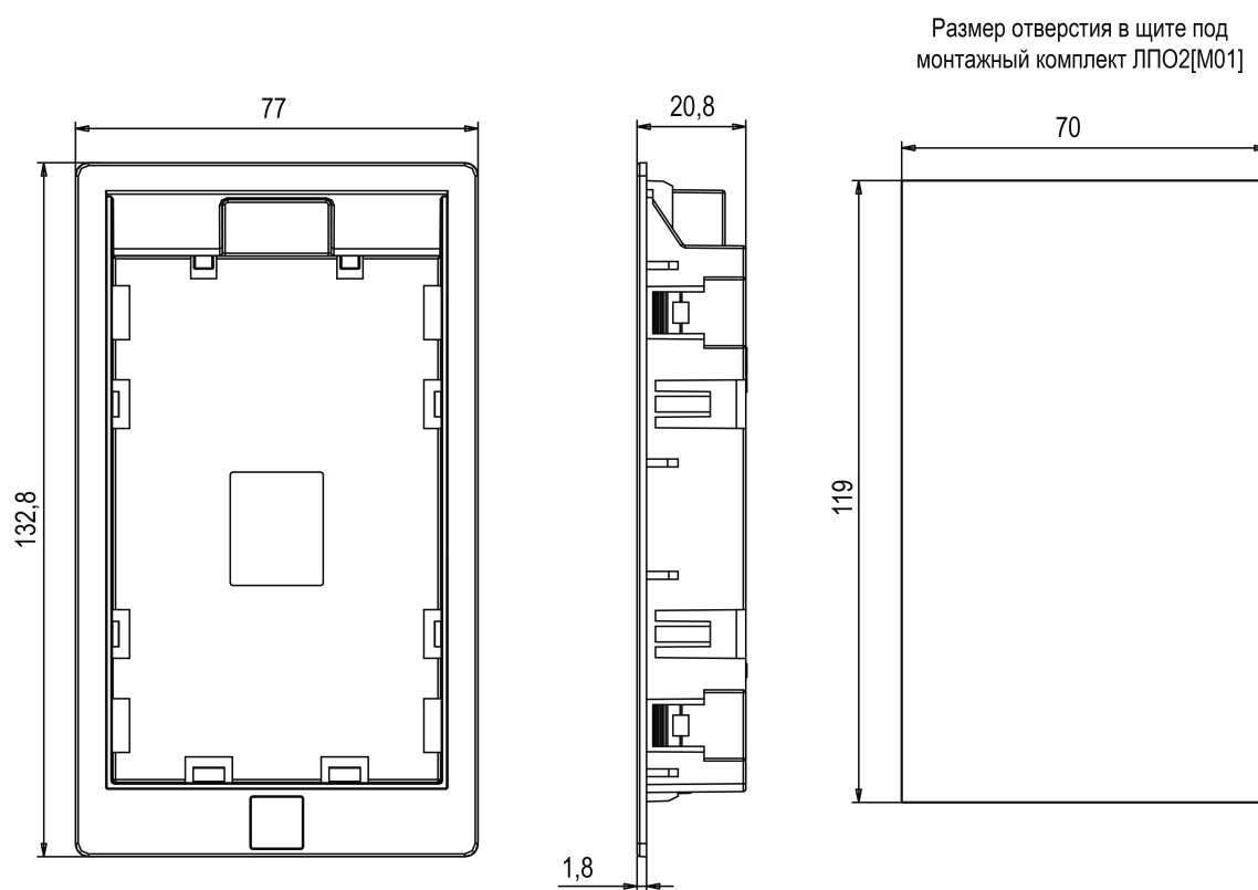
Рисунок 7.16 – Габаритные размеры комплекта для монтажа в щит ЛПО2(М01)
