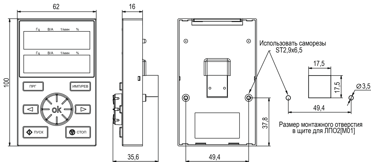
Рисунок 7.15 – Габаритные размеры внешней ЛПО2(M01)
