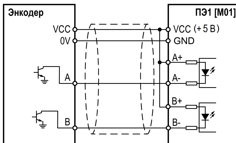
Рисунок 8.13 – Схема подключения энкодера с выходом типа «открытый коллектор»
