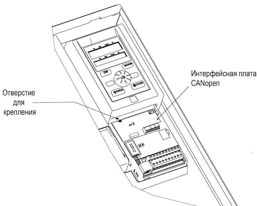
Рисунок 7.26 – Монтаж интерфейсной платы CANopen
