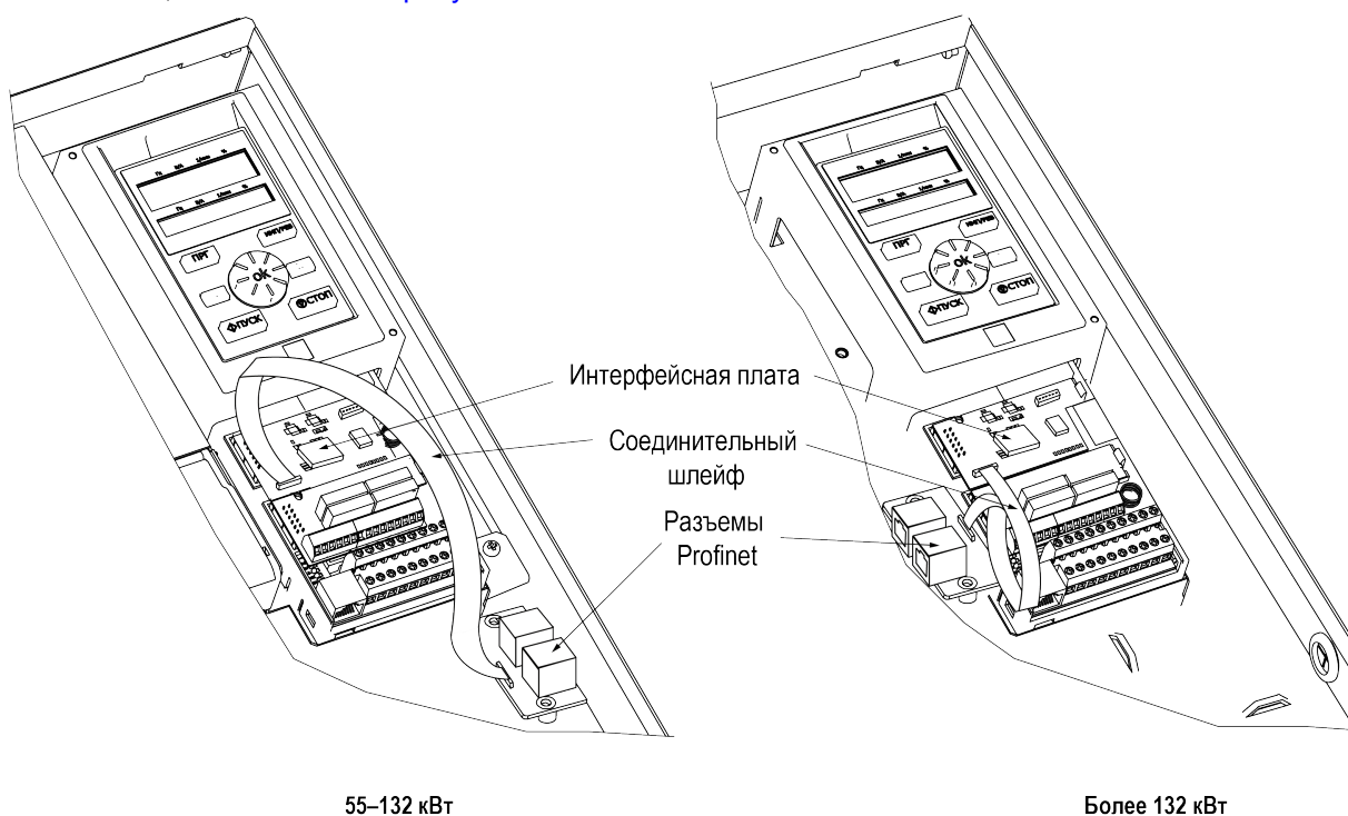
Рисунок 7.22 – Монтаж платы на преобразователях частоты мощностью более 45 кВт
