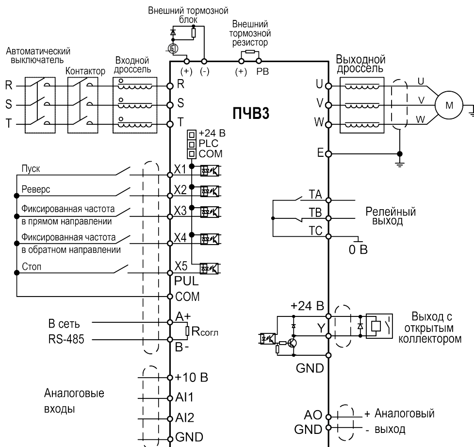
Рисунок 8.6 – Общая схема подключения
