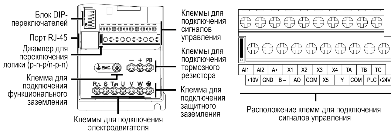
Рисунок 8.3 – Вид на клеммники (крышка снята)
