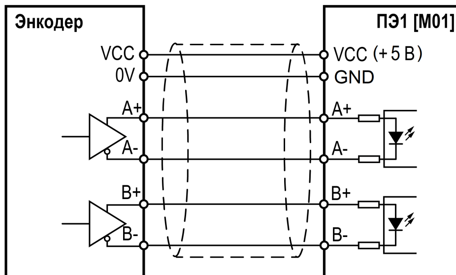
Рисунок 8.12 – Схема подключения энкодера с дифференциальным выходом
