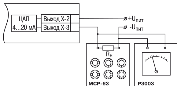
Рисунок 8.8 – Подключение ВУ1 типа И (R н =500 Ом)
