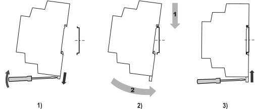
Рисунок 1 – Установка прибора
