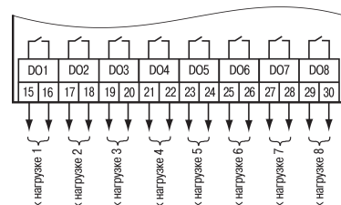
Рисунок 5 – Схема подключения нагрузки к ВЭ типа «Р»
