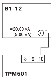
Рисунок 8.3 – Схема подключения
