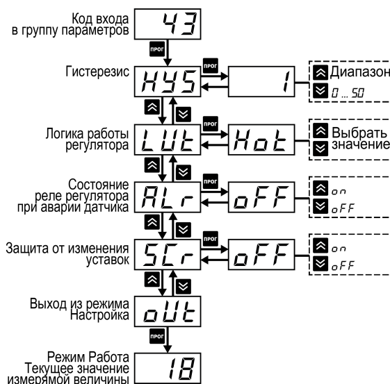
Рисунок 7.6 – Настройка параметров регулятора
