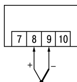
Рисунок 5.4 – Схема подключения ТП
