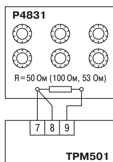
Рисунок 5.3 – Схема подключения
